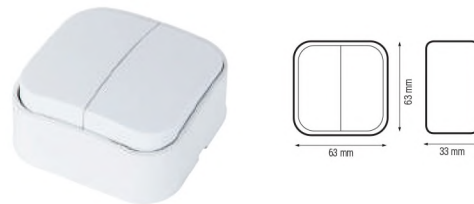
112 001 0003 ■ 2-GANG ONE WAY SWITCH (10A)
